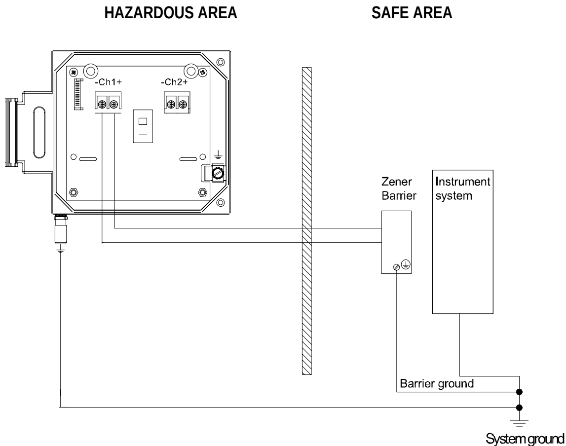
图 21 接地
