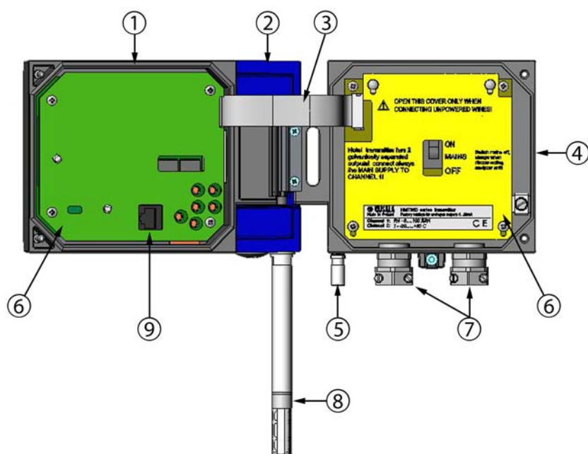
图7 变送器部件
